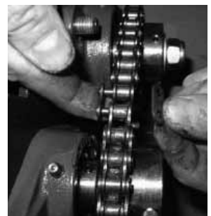
Kettengliedteil 2 positionieren
